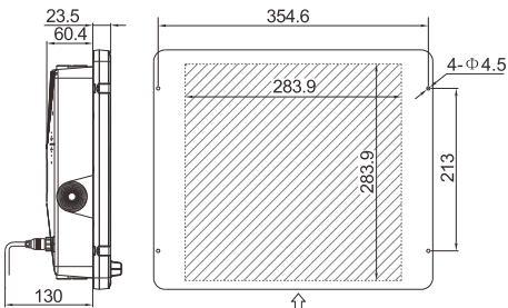
取孔尺寸圖
